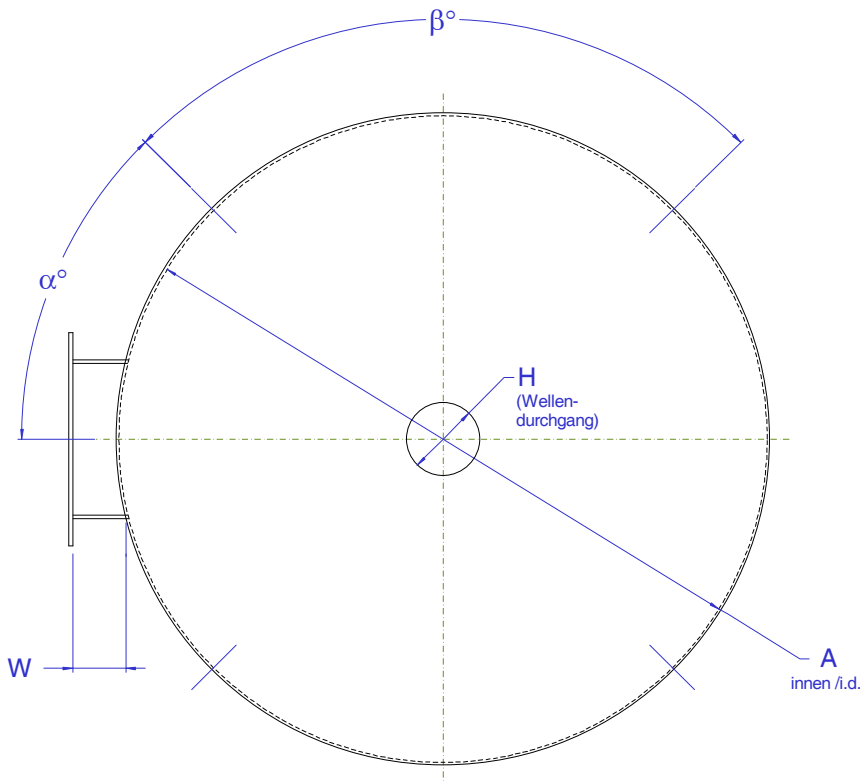
Abmessungen / Dimensions / Côtes
