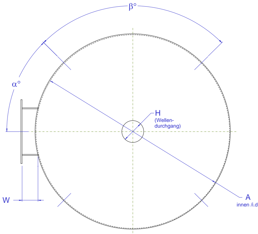
Abmessungen / Dimensions / Côtes
