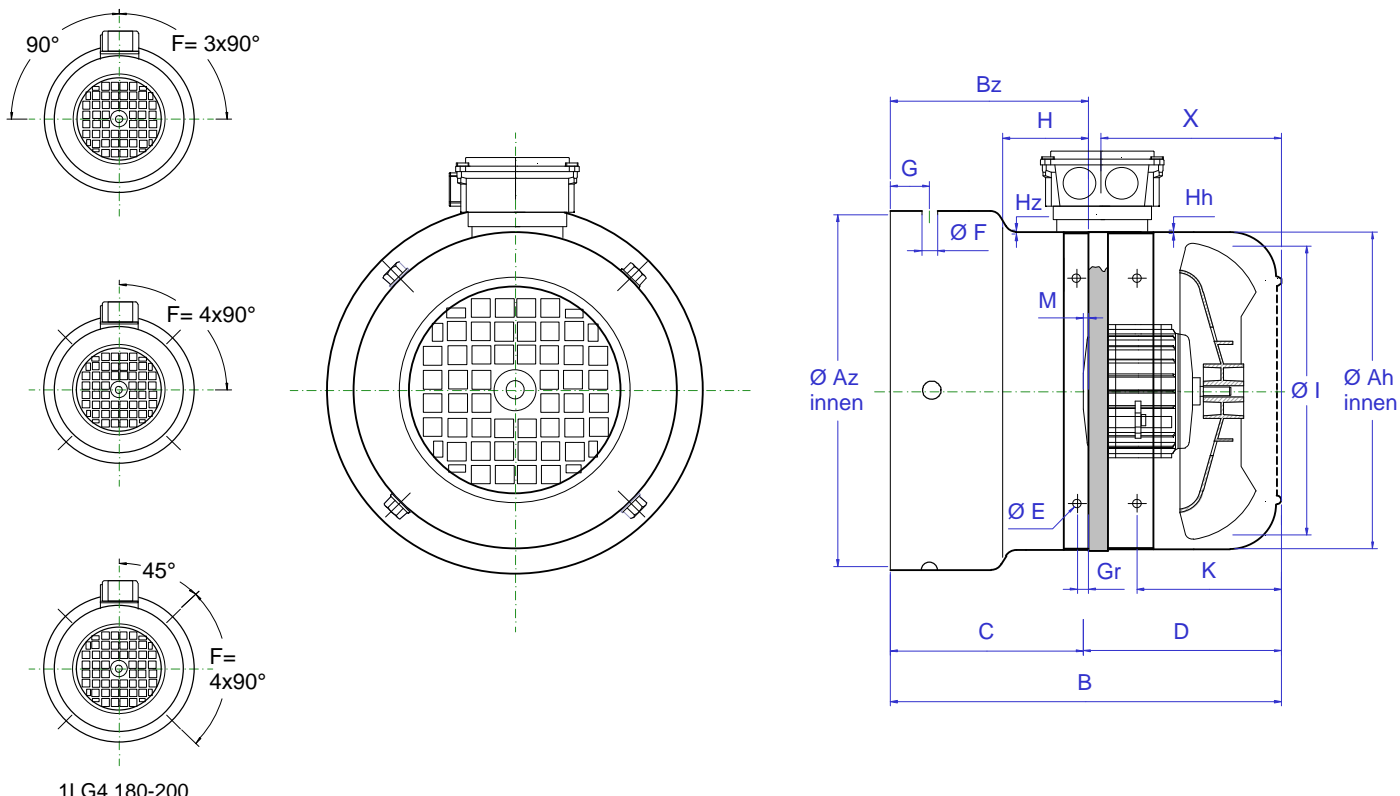
1LG4 180-200
