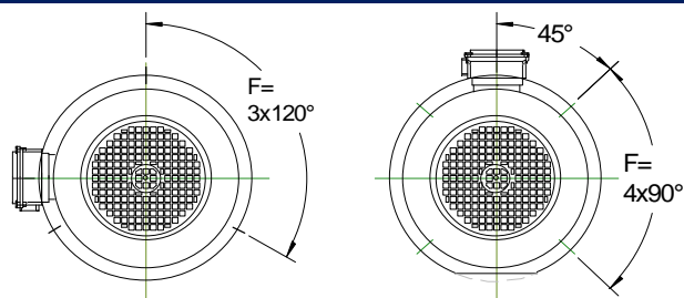
M2BA 132 - 225
