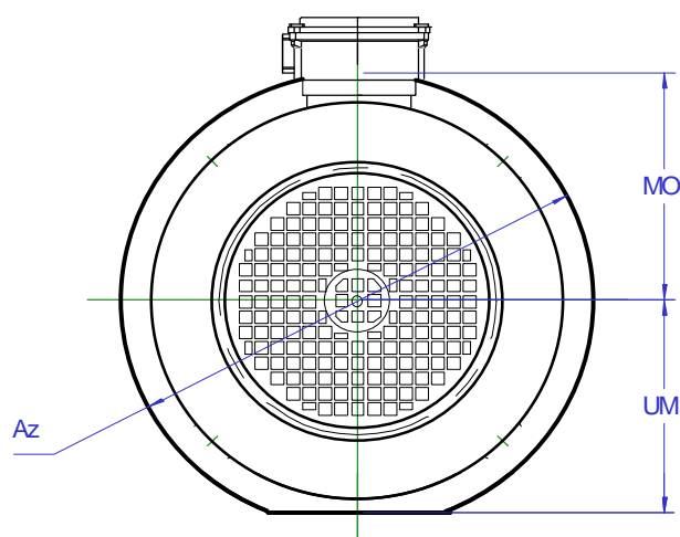
M2BA 80 - 112
